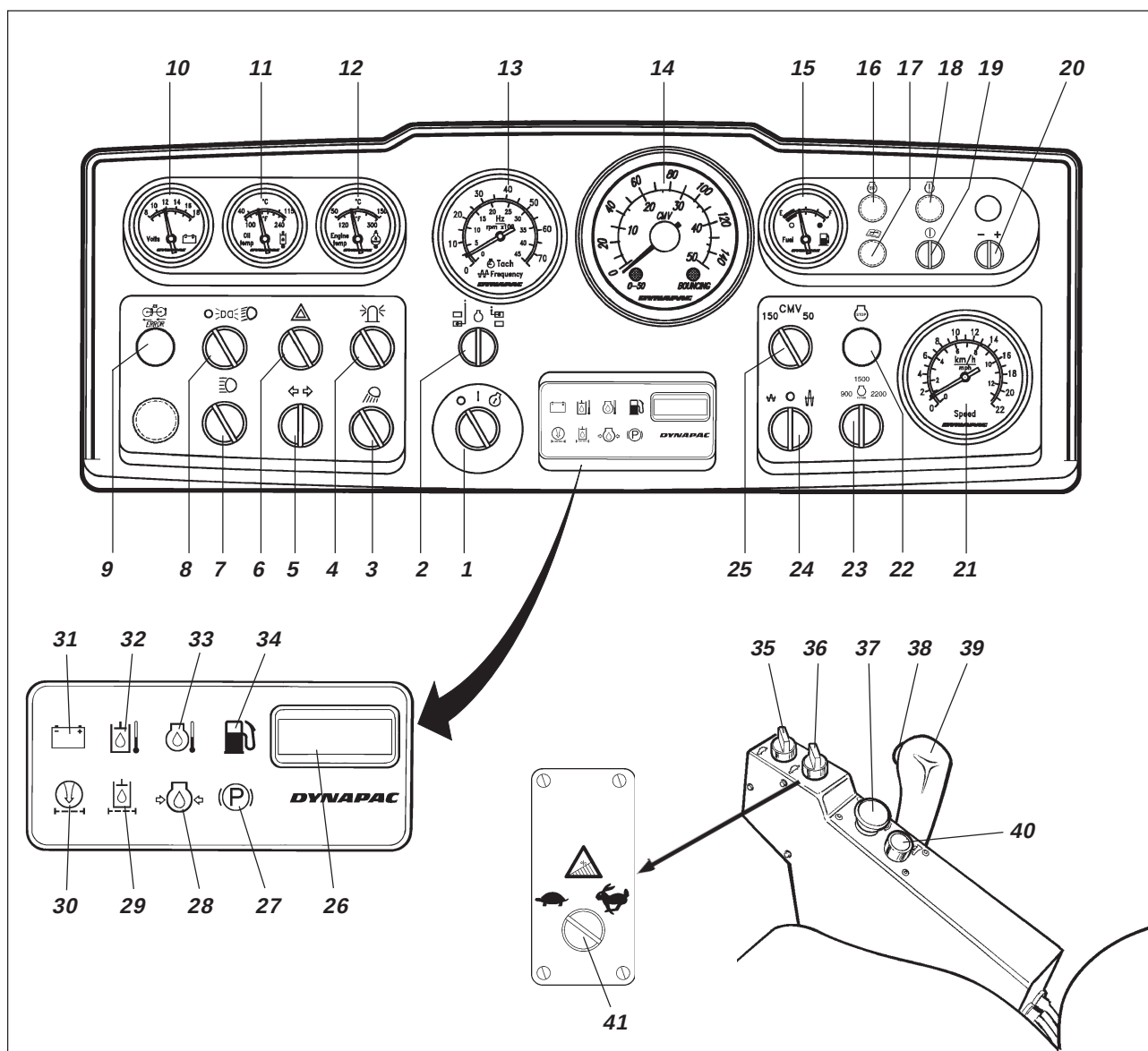
Fig. 7 Panneau d'instruments et commandes
