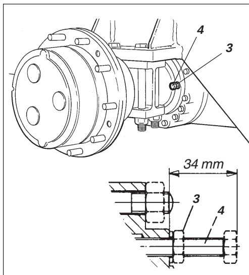
Fig. 34 Essieu arrière
