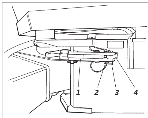
Fig. 32 Côté gauche de l'articulation centrale
