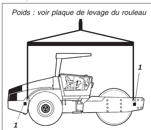
Fig. 31 Rouleau prêt au levage
