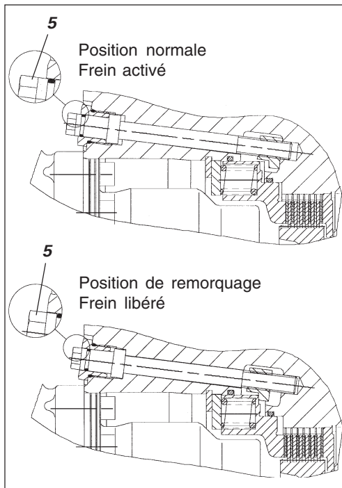
Fig. 35 Frein de cylindre 5. Vis
