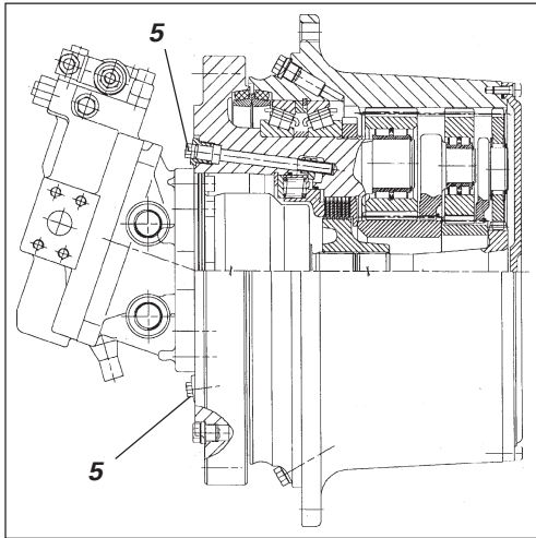
Fig. 35 Frein de cylindre 5. Vis
